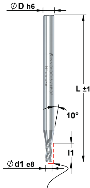
Zone de coupe Cutting edges (- - -)
